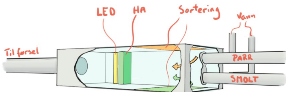
Figur 15: Rørskanner
